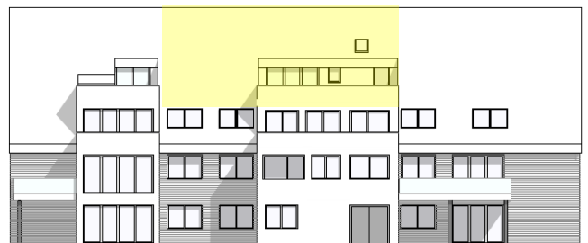
Ansicht Süd
